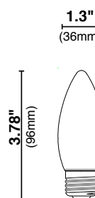
E26 B10
